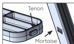
Double assemblage par tenon-mortaise + soudure
